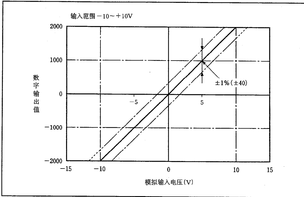
图3.3 电压输入特性的综合精度
