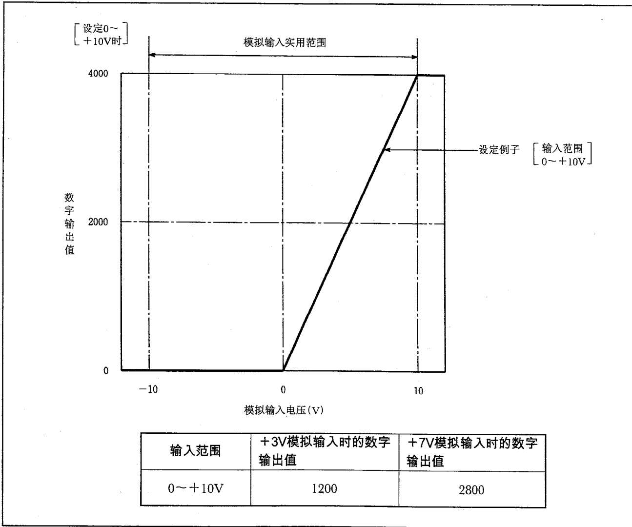
图3.1 电压输入特性
