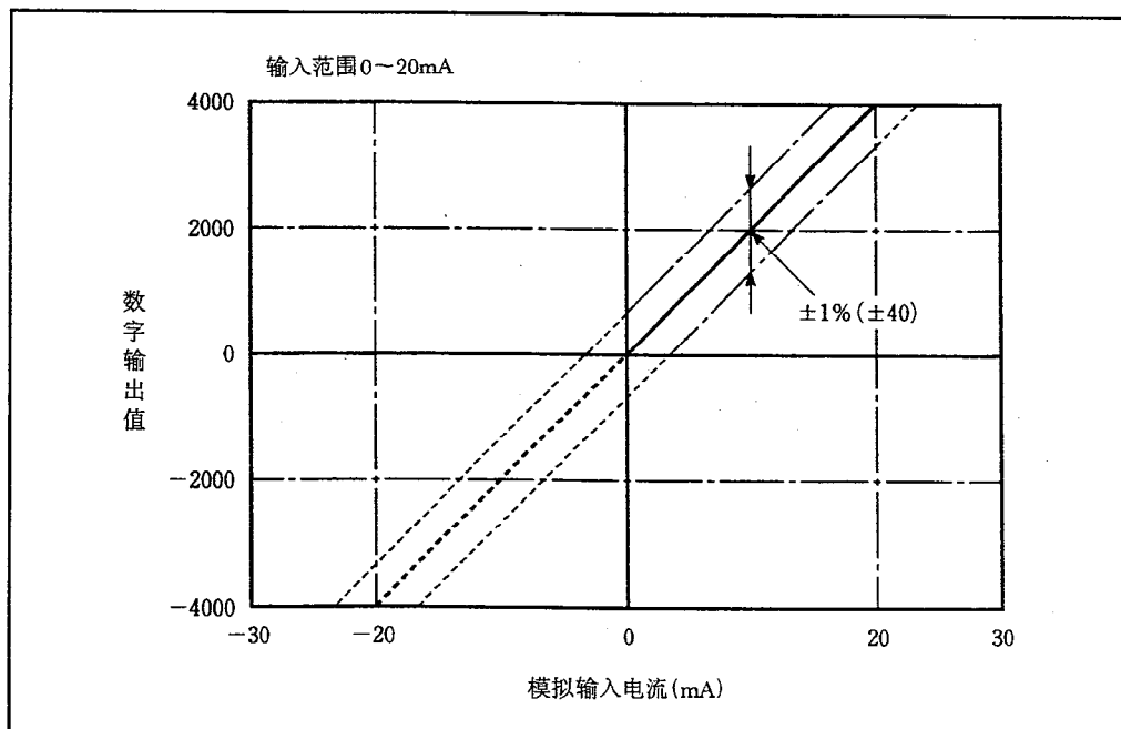
图3.4 电流输入特性的综合精度
