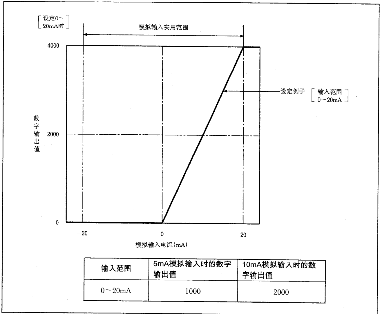
图3.3 电流输入特性
